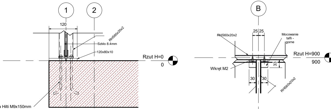
1 Mocowanie blachy 1 : 5
